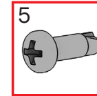
DIN 7504M-H 3,9x13
